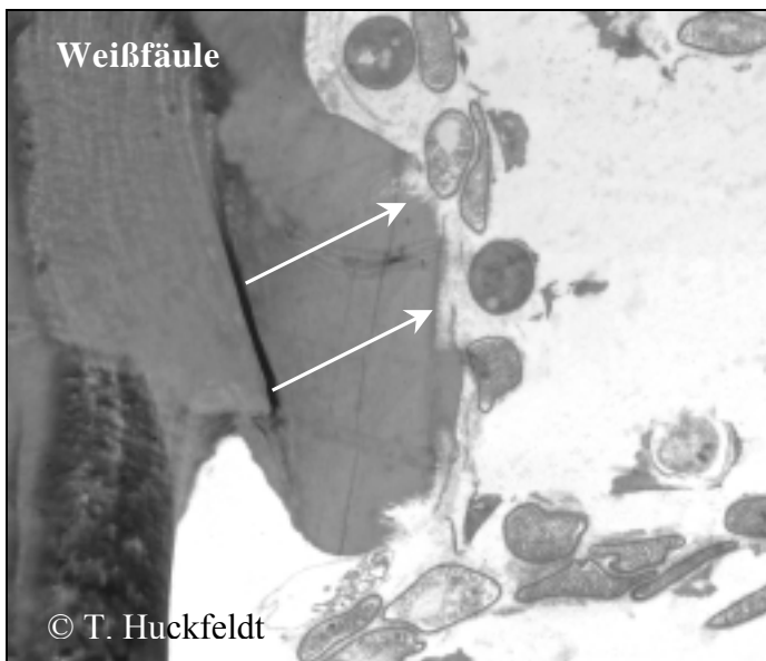
Abb. 4. Elektronenmikroskopische Aufnahme: Querschnitte von Hyphen des Ausgebreiteten Hausporlings ( Donkioporia expansa ), die im Holz liegen; die Zerstörung des Holzes verläuft streng von außen nach innen; der Abbau ist direkt unterhalb der Hyphen sichtbar (↑); Durchmesser der Hyphen ca. 1,5-3 \mu\text{m} .
